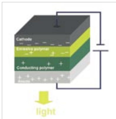
Funktionsweise eines OLED-Elements: Elektronenlöcher werden von der Anode und Elektronen von der Kathode emittiert. Im emissiven OLED-Polymer vereinigen sich Elektronenloch und Elektron und emittieren Licht.
