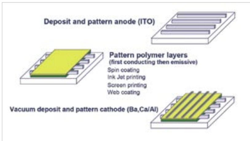
Schema des räumlichen Aufbaus bei der Herstellung eines OLED-Displays.
