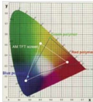
Der Farbraum der spektralen Emission eines OLED-Displays im Vergleich zum verbreiteten TFT-Display.
