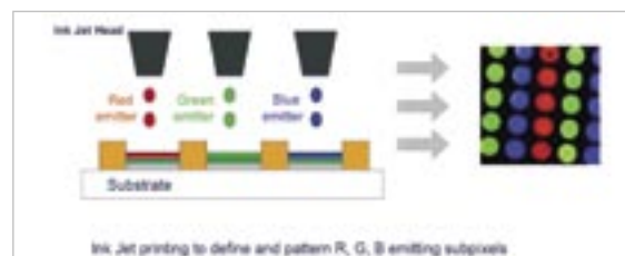
Die Inkjet Print-Methode ist ein aussichtsreiches und sehr präzises Verfahren zur Applikation der einzelnen Farbpixel bei der Herstellung eines OLED-Displays.
