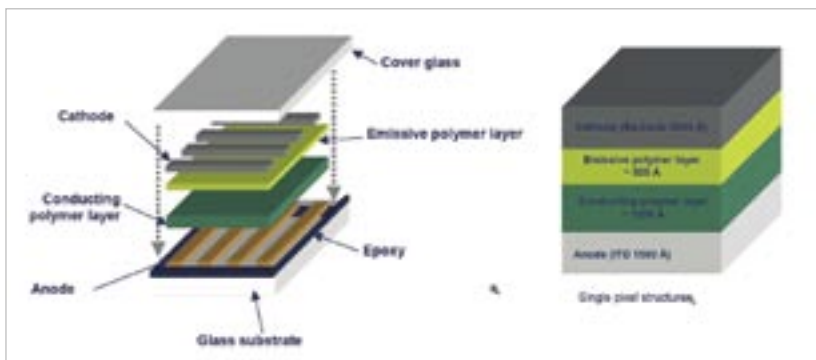
Aufbau und Struktur des OLED-Displays und eines einzelnen Pixels.
